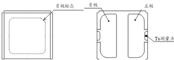
图2 T_S 测量点 (NVSU233C)
