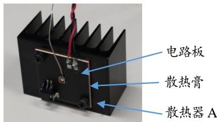
照片 3 评价光源的散热结构 (NVSU233C)
