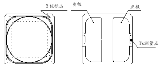
图3 T_S 测量点 (NVSU233C-D4)
