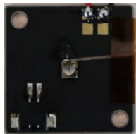
照片 2 安装状态 (NVSU233C-D4)
