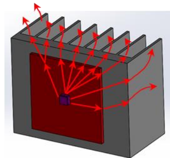
图 5 让鳍片向侧面设置时的 散热路径示意图
