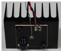
照片 5 让鳍片向侧面设置 (日亚设置朝向)
