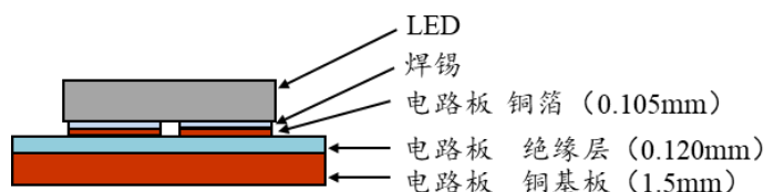
图 4 电路板安装时结构
