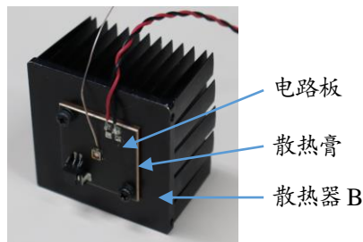
照片 4 评价光源的散热结构 (NVSU233C)
